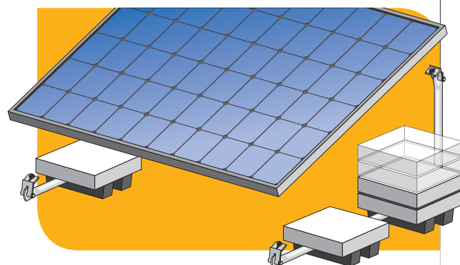
De ValkBox 3 (platte daken) bevat een duidelijke ballast-tabel met windregio- en gebouwhoogte-variabelen, waarmee u snel de juiste verzwarende kunt bepalen.
